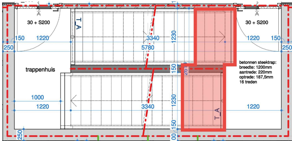
Extra ruimte appartement bij lagere plafondhoogte (rode kader)
